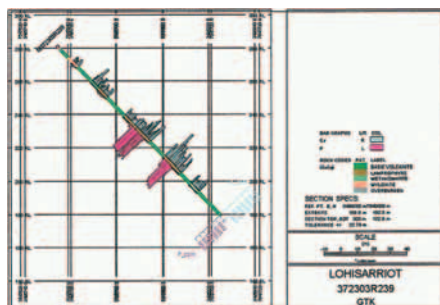
Kuva 10. Fosforin (P) ja kalsiumin (Ca) pitoisuudet syväkaira-reiässä R239.
