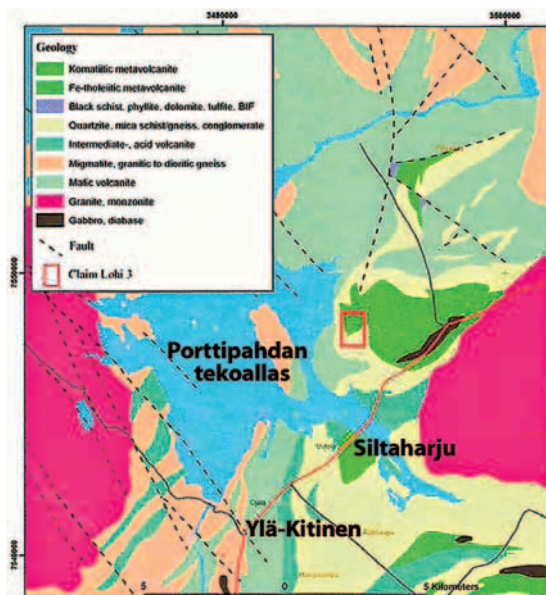
Kuva 2. Lohisarrioiden sijoittuvat Ruosselän graniittikompleksin länsi kontaktiin (Lehtonen et al. 1998).
