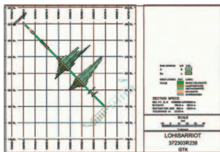
Kuva 9. Bariumin (Ba) ja kaliumin (K) pitoisuudet syväkaira-reiässä R239.
