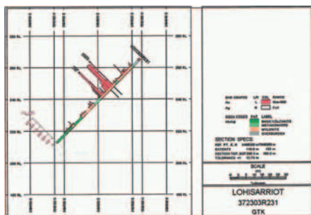
Kuva 7. Kulta- ja kuparipitoisuus syväkaira-reiässä R231.
