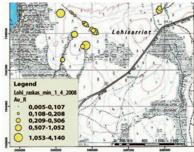
Kuva 4. Lohisarrioiden ensimmäisen raskasmineraalitutkimuksen hippukartta.
