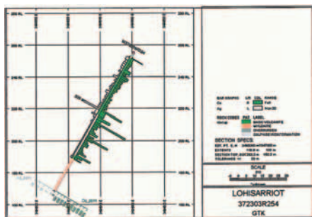
Kuva 6. Hopea- ja kuparipitoisuus koekaira-reiässä R254.
