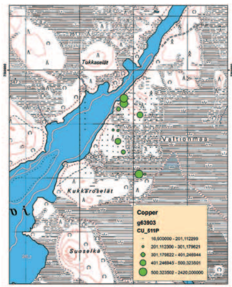
Kuva 4. Moreenin kuparipitoisuus Kukkaro selässä.
