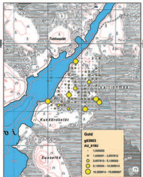
Kuva 2. Moreenin kultapitoisuus Kukkaroselässä.
