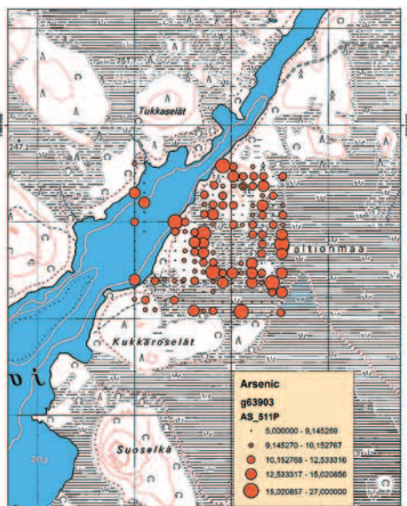
Kuva 3. Moreenin arseenipitoisuus Kukkaroselässä.
