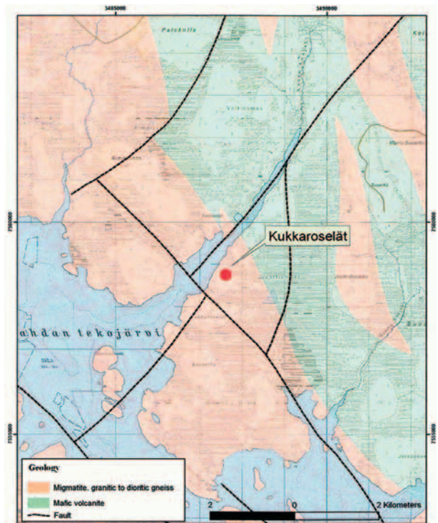
Kuva 1. Kukkaroselän sijainti ja kallioperäkartta
