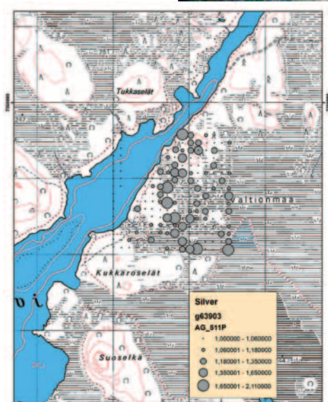
Kuva 5. Moreenin hopeapitoisuus Kukkaro selässä.
