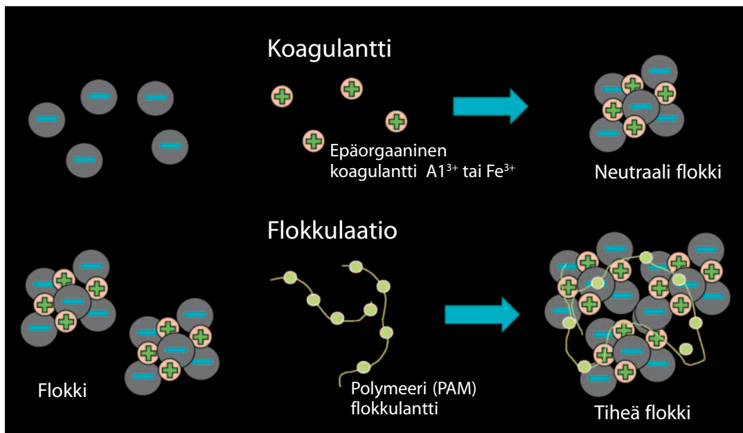
Koagulantin ja flokkulantin hahmollistettava kaavio.
