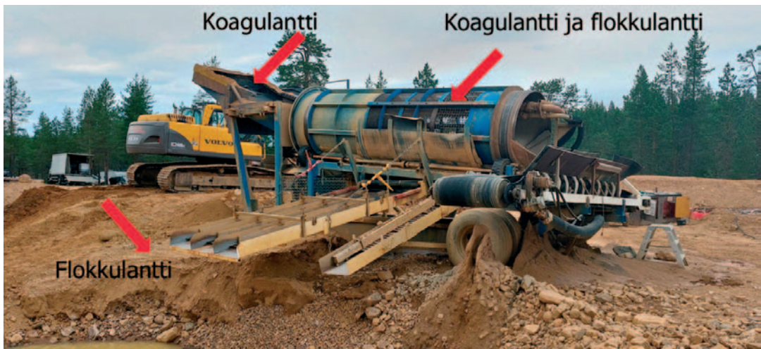
Jaskarin erottelulaite, Selperin testeille. Kuva: Esther Takaluoma
