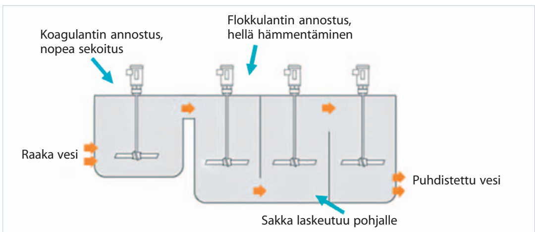
Sekoitus ja laskeuttamisaltaat teollisuuskäytössä, kaavio.
