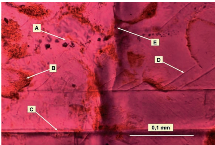
Polarisaatiomikroskooppikuva Puskun pinkistä safiirista läpikulkevassa valossa. A. Sekundaareja fluidisulkeumia mikrohalkeamissa. B. Rautaoksihydraattia ja savimineraaleja pinnan koloissa. C. Korundille tyypillisiä jakautumapintoja. D. Jännityshalkeamia. E. Jäätikkö- tai jokikuljetuksessa syntyneitä mikrohalkeamia. Kuva: Kari A. Kinnunen.
